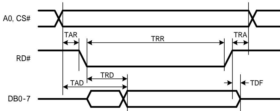
図 7-1) CPU読み出しタイミング
