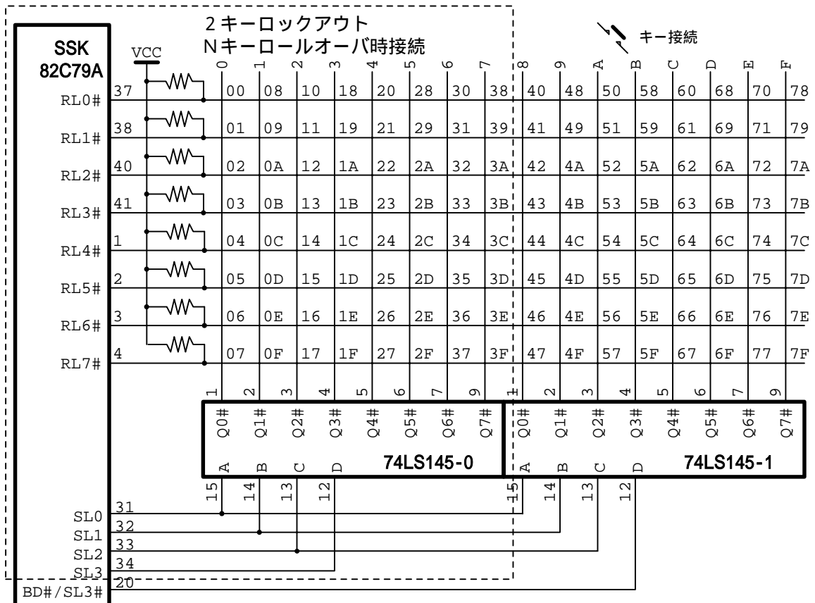
図 3-4) キー接続例
