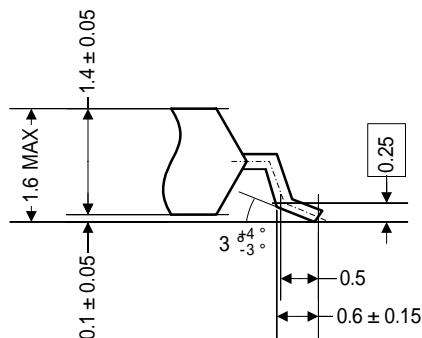
端子先端詳細図
