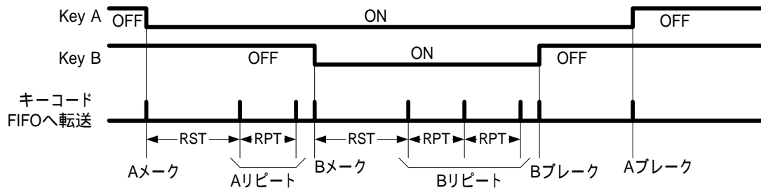
図 3-4) キー接続例
