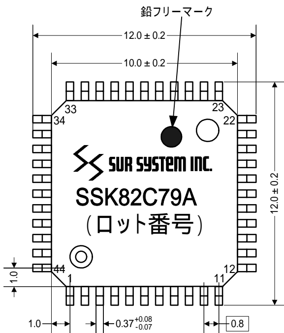
図 7-5) SSK82C79A 外形・捺印図
