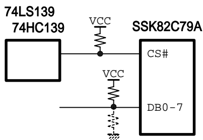
図 6-1) CMOS レベルへの変更
